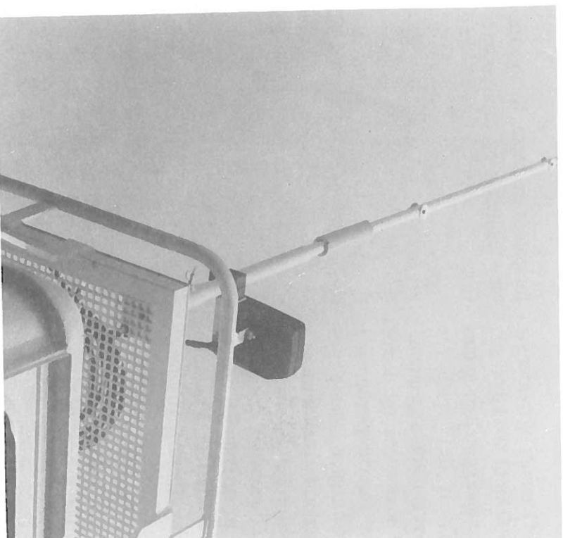
Det Nye flagholdersystem i nærhillede, her monteret på Magirus 178, som i forvejen er høj FOTO: PGS
